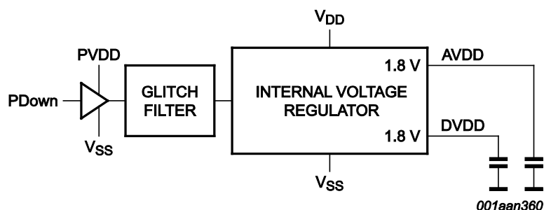
图 33. 内部 PDown 到电压调节器逻辑
