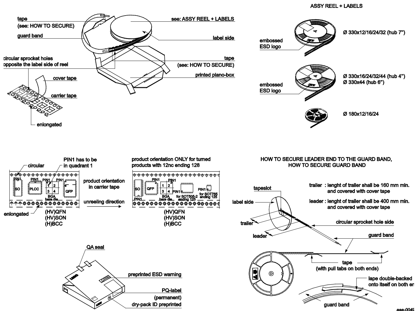
图 41. 卷轴封装信息
