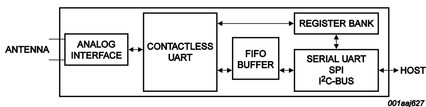
图 1. CLRC663 简化框图
