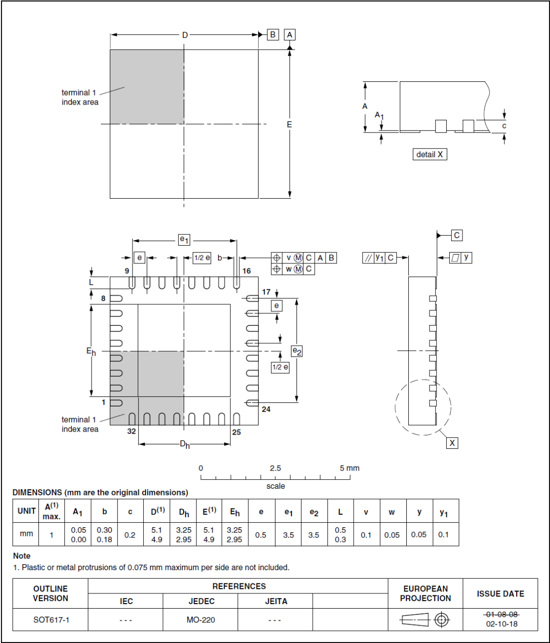
图 37. SOT617-1（HVQFN32）封装
