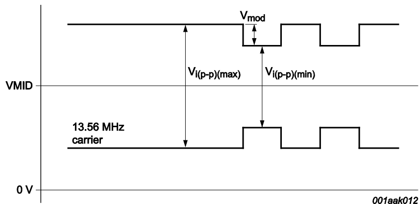
图 34. RX 引脚输入电压
