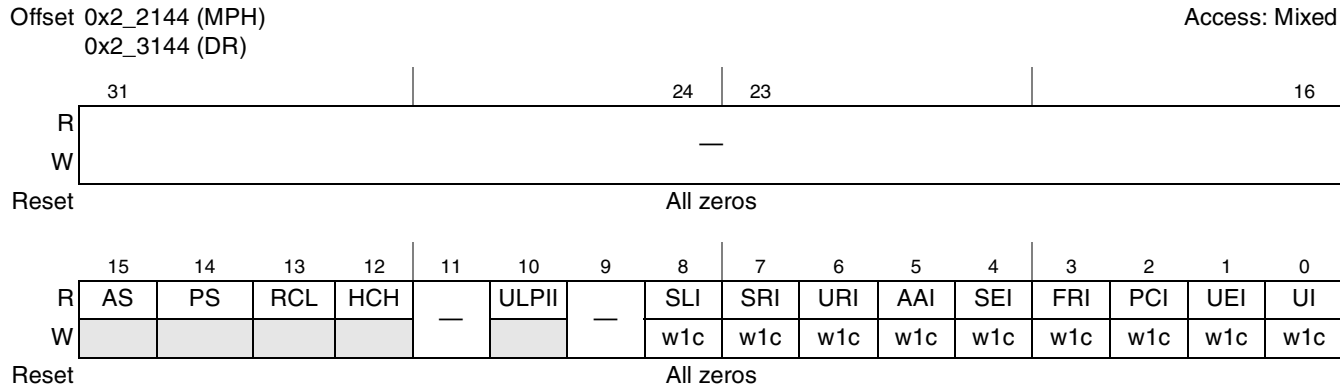
Figure 16-9. USB Status Register (USBSTS)
