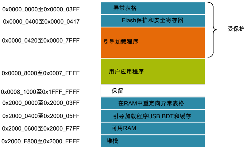
图 1. ColdFire V2 引导加载程序存储器映射
