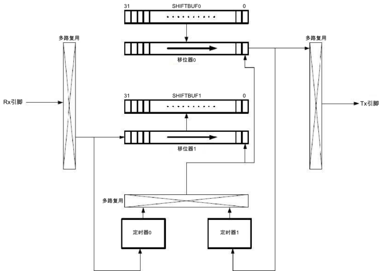
图 2. UART 模拟框图
