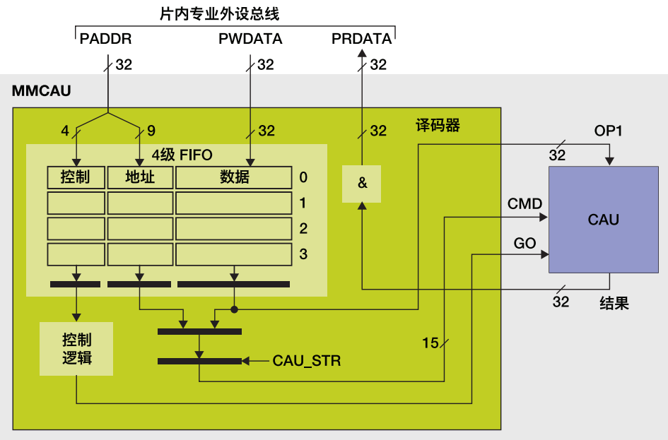
MMCAU框图
