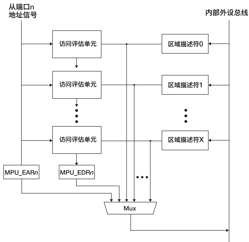
存储器保护单元框图
